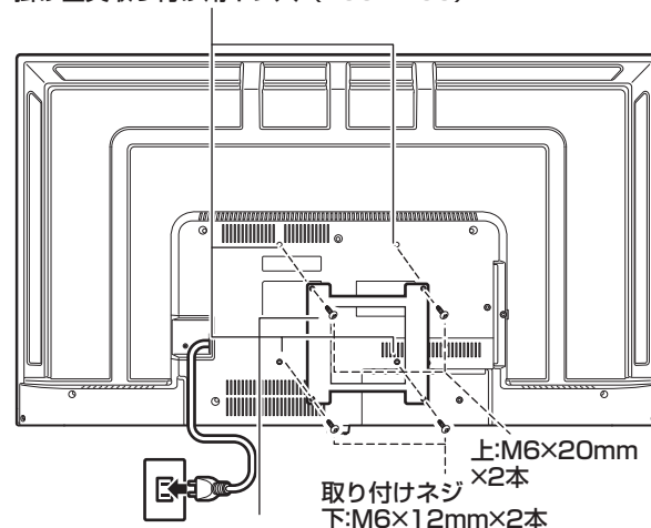
掛け金具取り付け用ネジ穴 (200×200)
